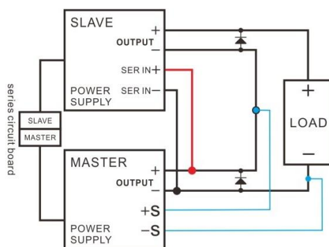
图 5-2 串联模式远端补偿接线
