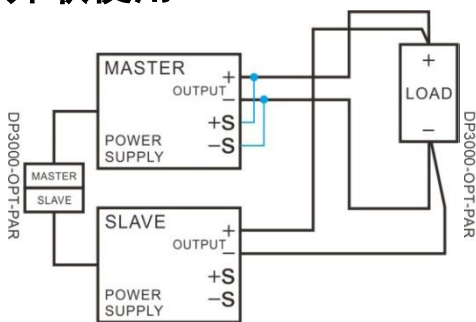
图 5-3 两台并联时，近端补偿接线
