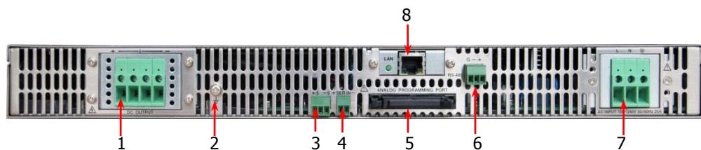
图 1-2 后面板
