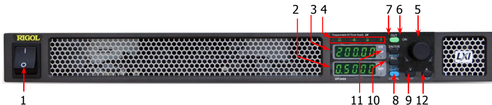
图 1-1 前面板
