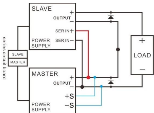
图 5-1 (LOCAL) 串联模式近端补偿接线
