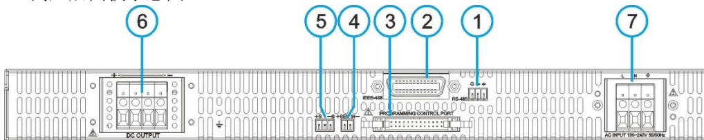
1U 高压后面板示意图 (150V~600V models)
