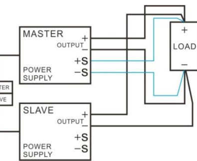
图 5-4 两台并联时，远端补偿接线
