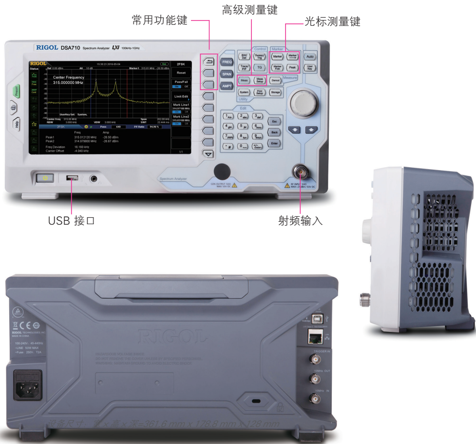
设备尺寸: 宽×高×深=361.6 mm x 178.8 mm x 128 mm
